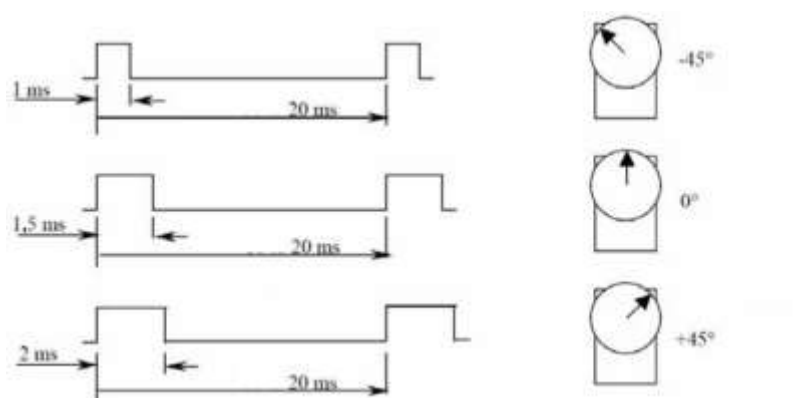
3 pav. Mechanizmo valdymo signalas
