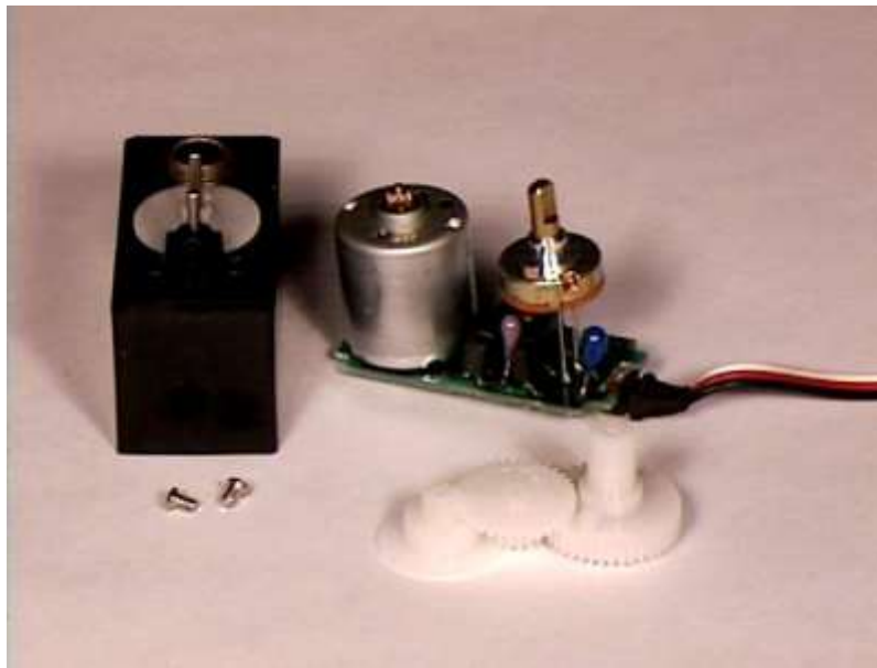
2 pav. Išardytas valdomasis mechanizmas (Seattle Robotics Society nuotrauka)
